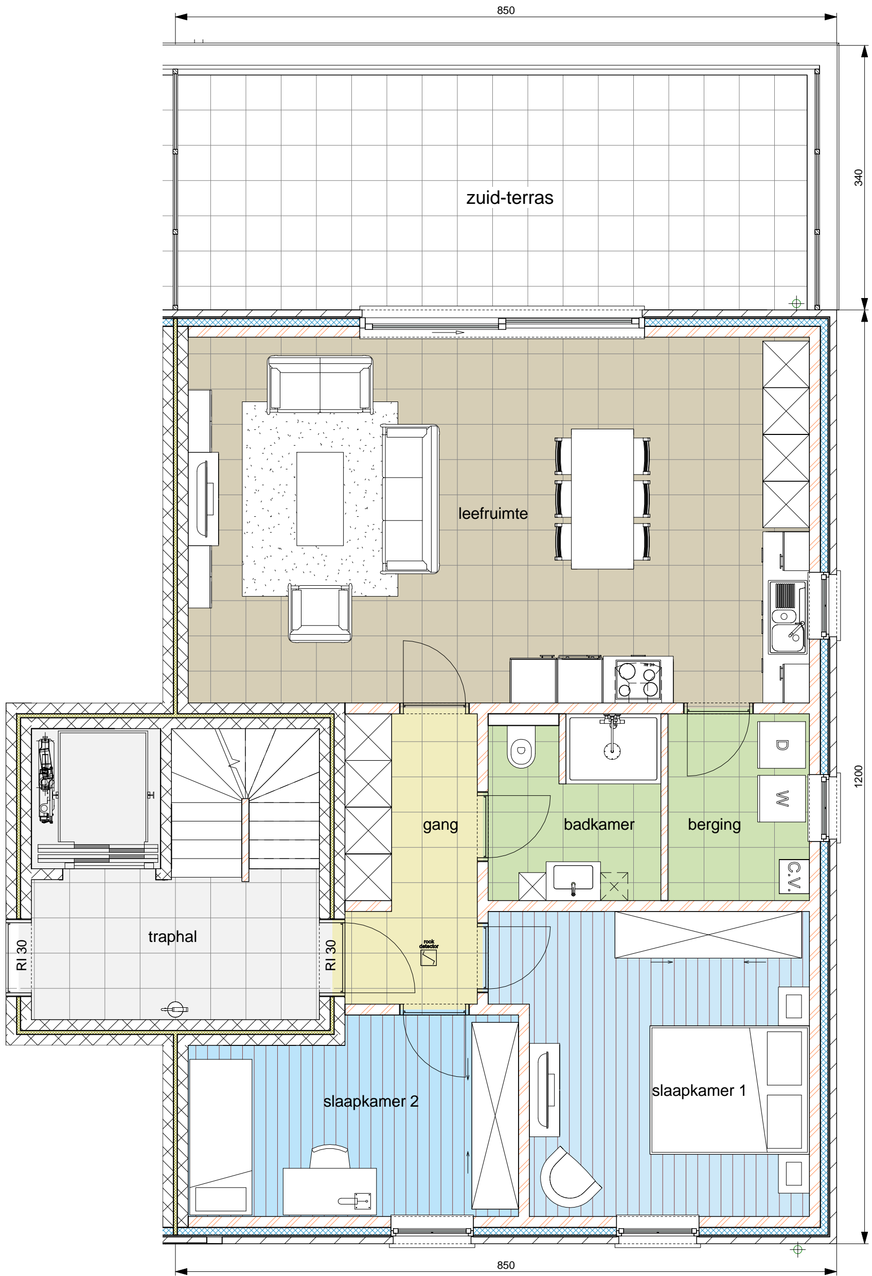
8 Appartement 08 1 : 50
