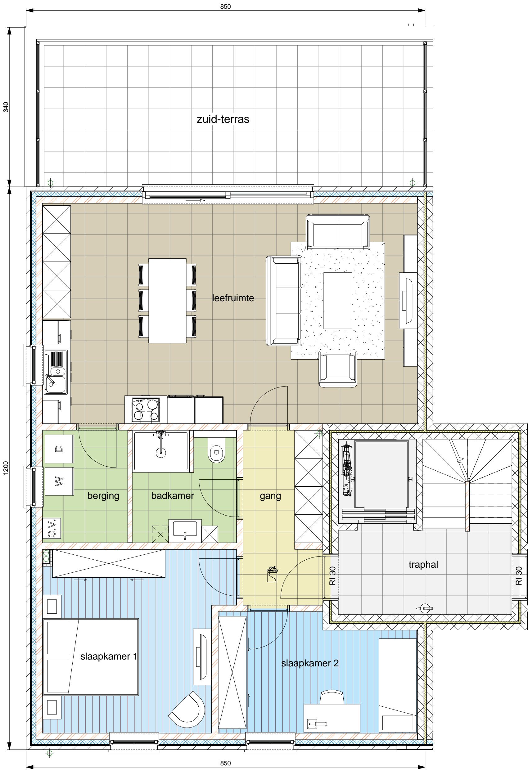
7 Appartement 07 1 : 50
