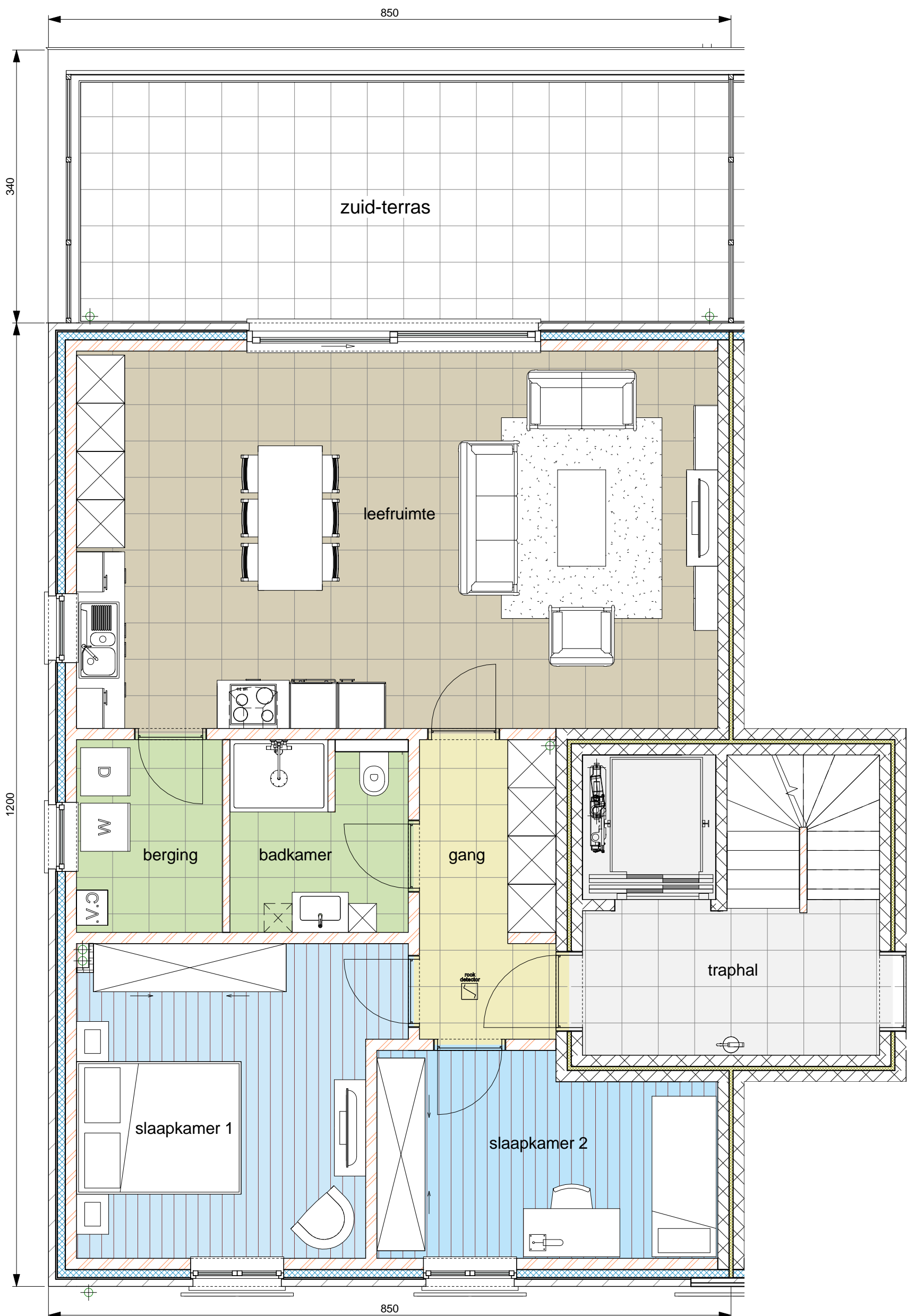
5 Appartement 05 1 : 50
